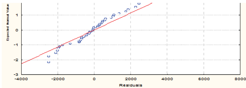
Рис. 1. График остатков регрессии для первого кластера
