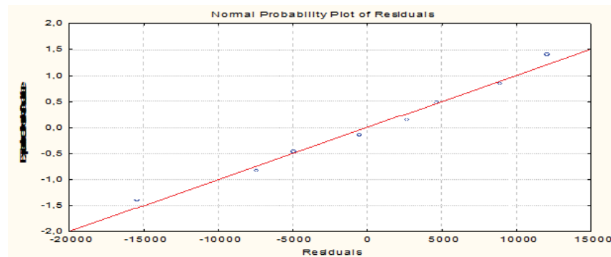
Рис. 3. Нормальный график остатков регрессии для третьего кластера
