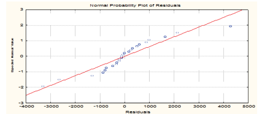
Рис. 2. График остатков регрессии для второго кластера
